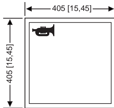
frontale - sez. altoparlante
